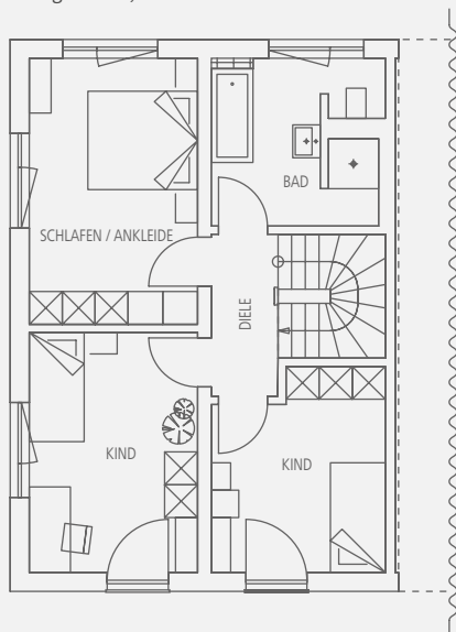
Obergeschoss, ca. 52 m 2 NGF.
