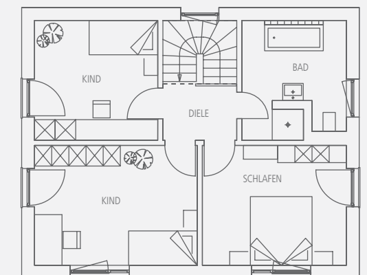
Obergeschoss, ca. 57 m 2 NGF.
