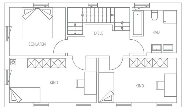
Obergeschoss, ca. 64 m 2 WF.
