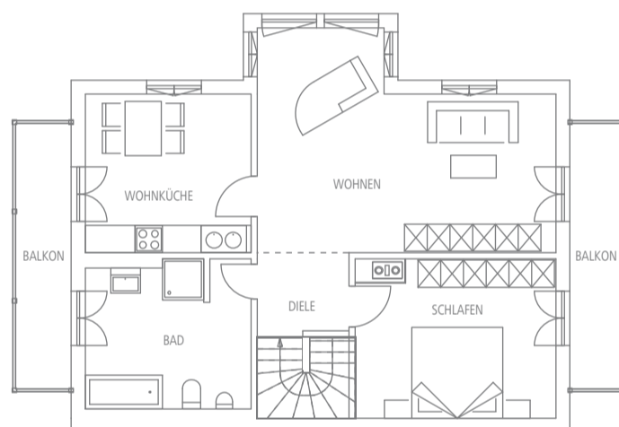
Obergeschoss, ca. 73 m 2 WF.
